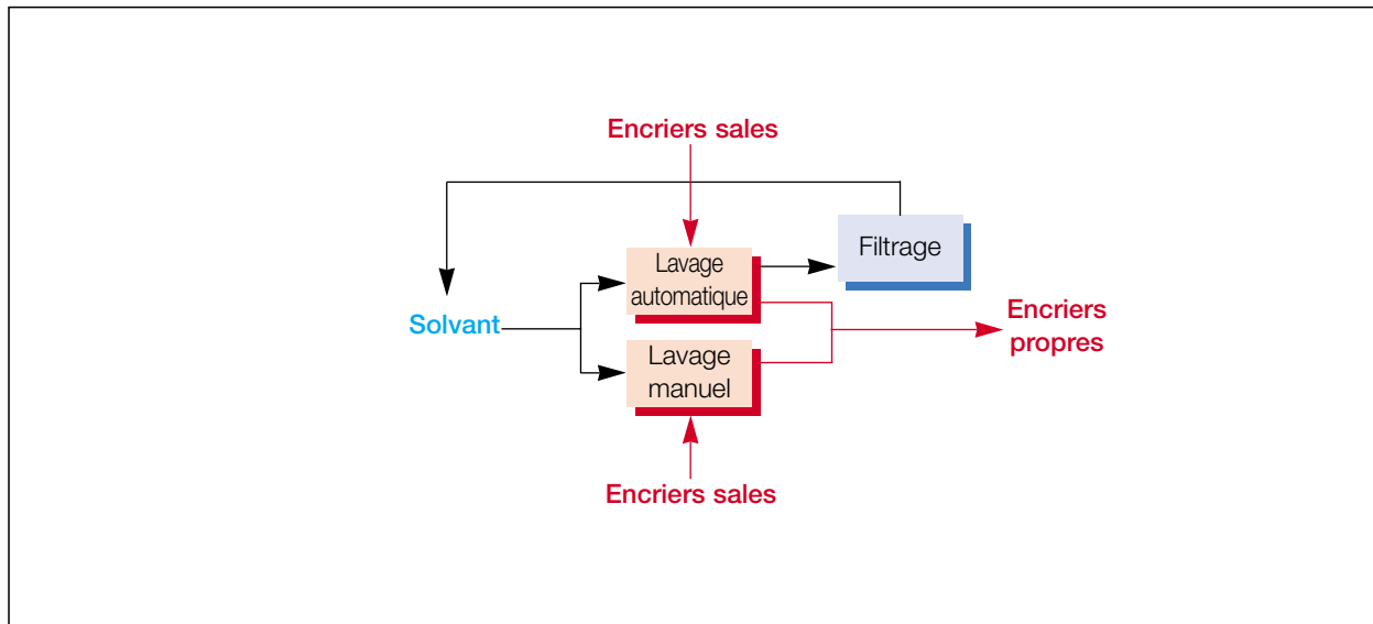
Figure 15 DIAGRAMME DU PROCÉDÉ DE NETTOYAGE DE L'ENTREPRISE TOTALPACK
