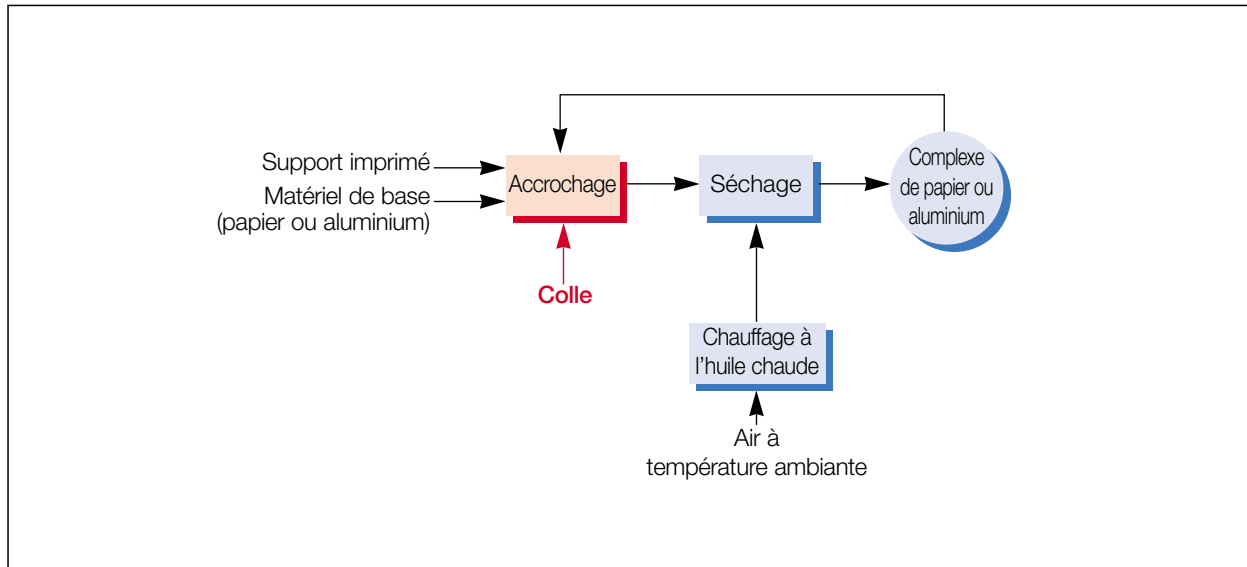
Figure 14 DIAGRAMME DU PROCÉDÉ DE LAMINAGE DE L'ENTREPRISE TOTALPACK
