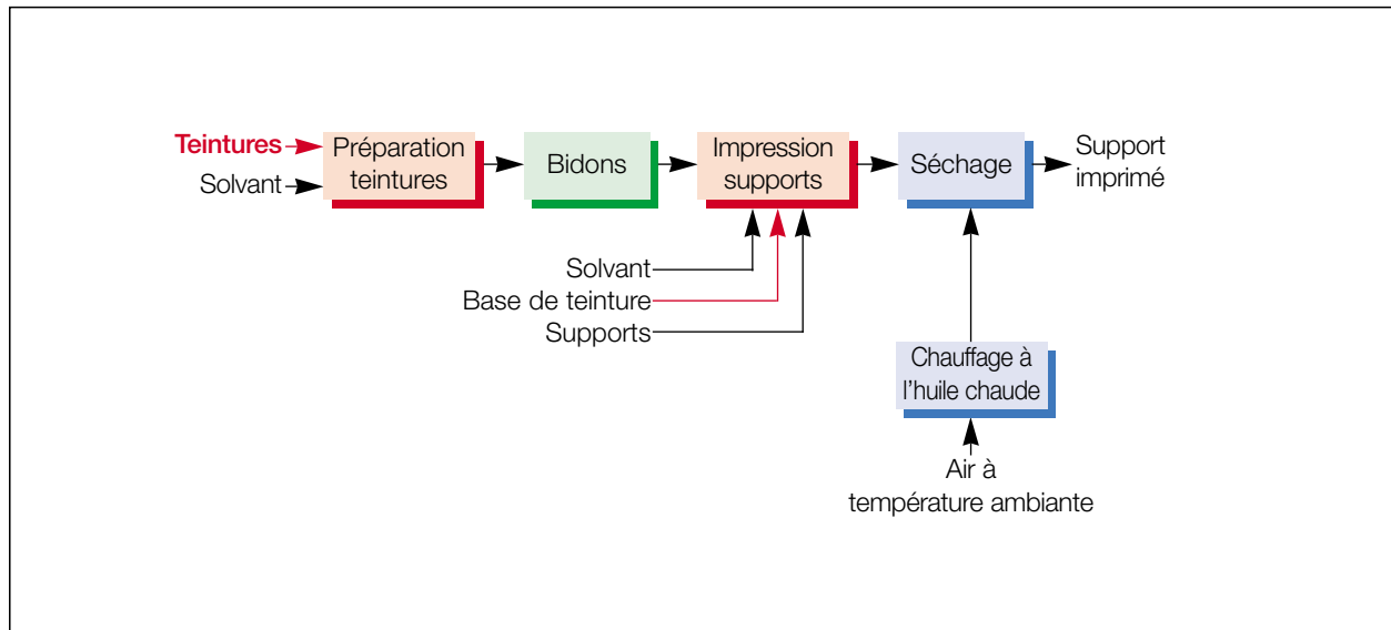
Figure 13 DIAGRAMME DU PROCÉDÉ D'IMPRESSION DE L'ENTREPRISE TOTALPACK
