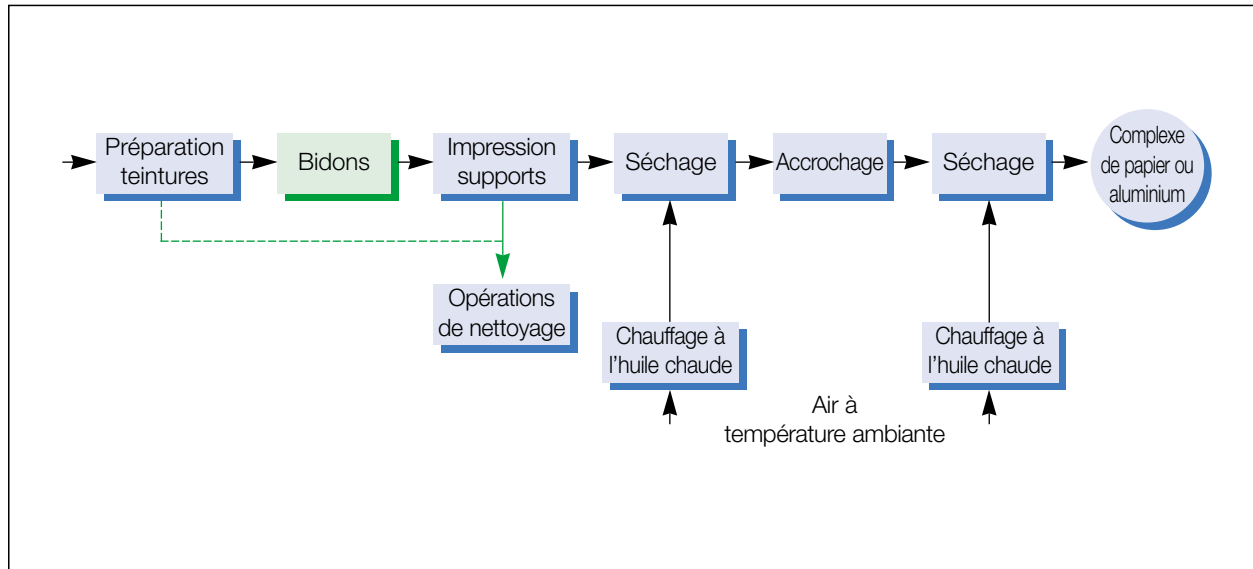
Figure 12 DIAGRAMME DU PROCÉDÉ DE L'ENTREPRISE TOTALPACK
